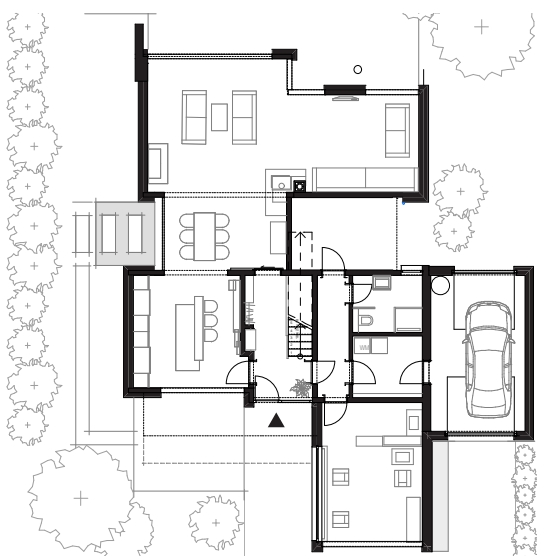
Haus K_4. Grundrisse.
