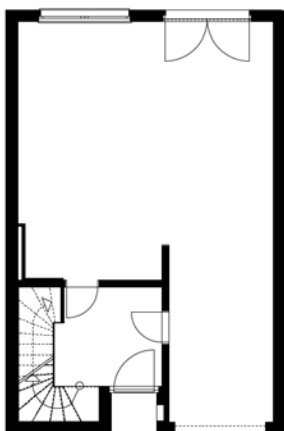
Eisenacher Straße. Grundrisse.
